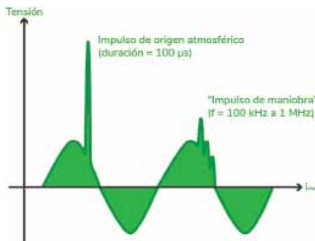
Sobretensiones transitorias
